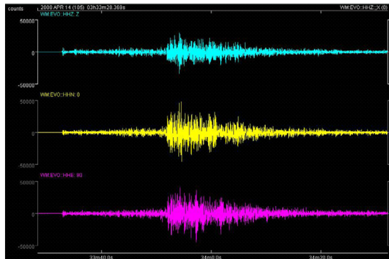
Registo do sismo do 14 de Abril de 2008 - Estação EVO ( Centro de Geofísica de Évora )
