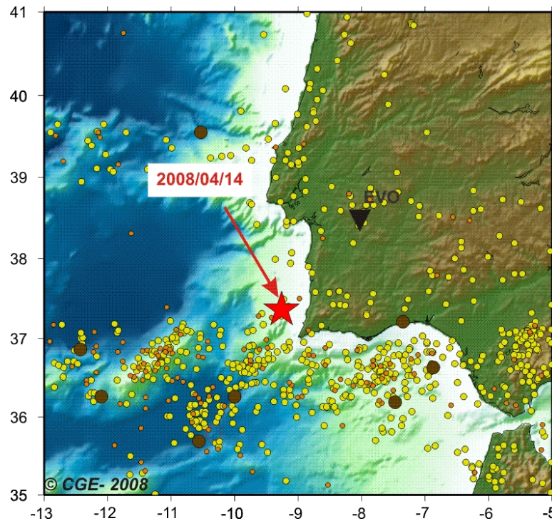
Sismicidade da Zona Sul de Portugal com destaque para o sismo do 14 de Abril de 2008 (Magnitude – informação do Instituto de Meteorologia)
